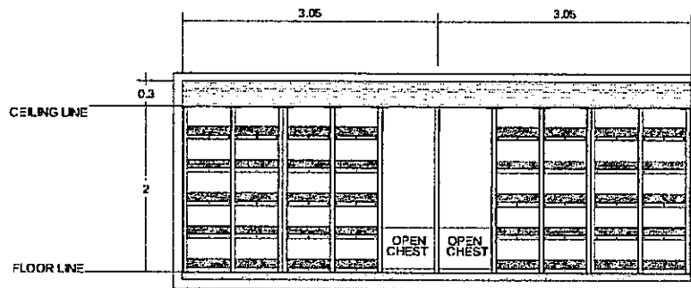
LONGITUDINAL SECTION
